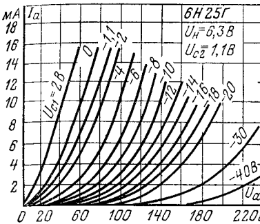
Анодные характеристики.
