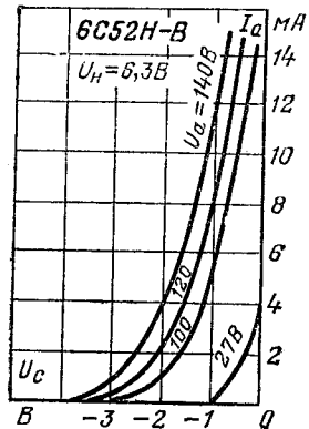
Анодно-сеточные характеристики.
