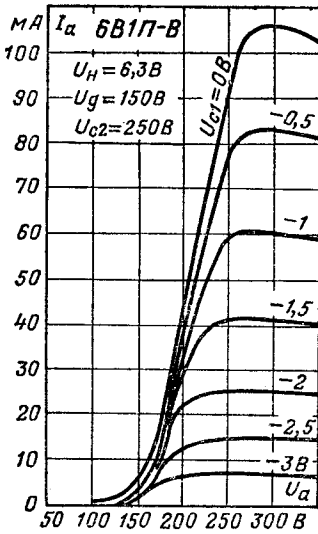
Анодные характеристики.
