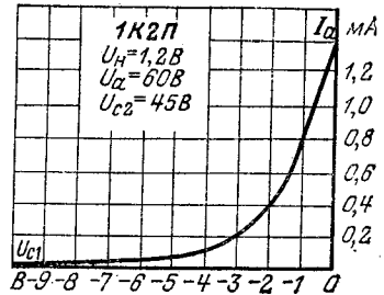
Анодно-сеточные характеристики.
