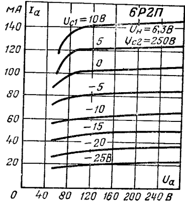
Анодные характеристики.
