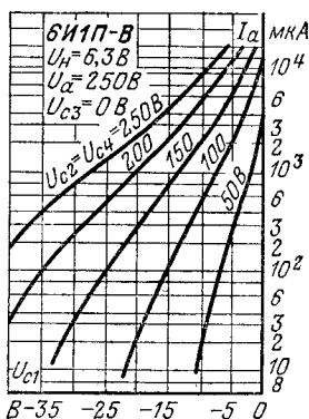
Анодно-сеточные характеристики геттодной части.
