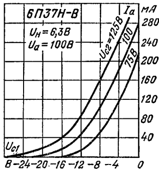
Анодно-сеточные характеристики.
