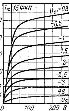
Анодные характеристики пентодной части.
