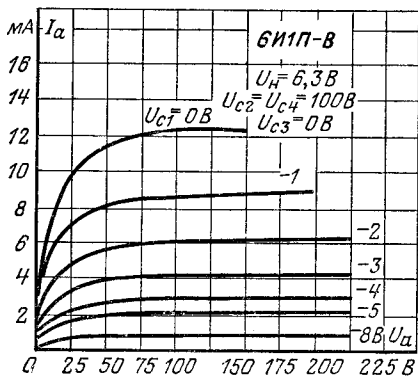
Анодные характеристики геттодной части.
