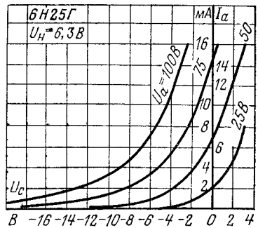
Анодно-сеточные характеристики.
