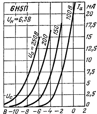
Анодно-сеточные характеристики.
