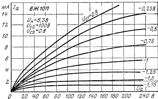
Анодные характеристики.
