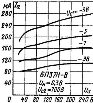
Анодные характеристики.
