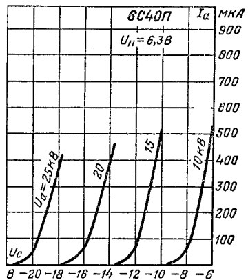
Анодно-сеточные характеристики.
