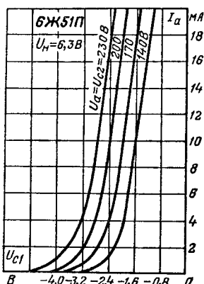
Анодно-сеточные характеристики.
