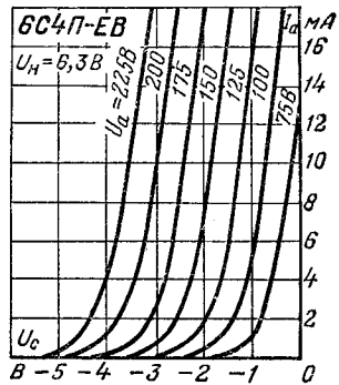
Анодно-сеточные характеристики.
