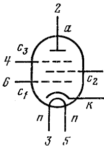
6Ж10Б-ВР
